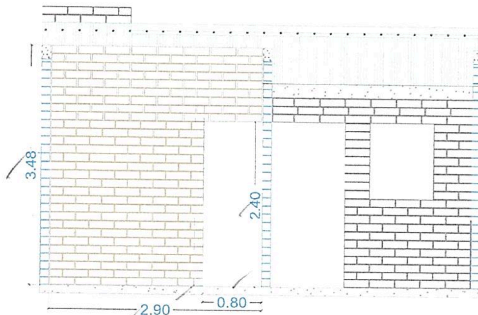
MURO EJE 3
