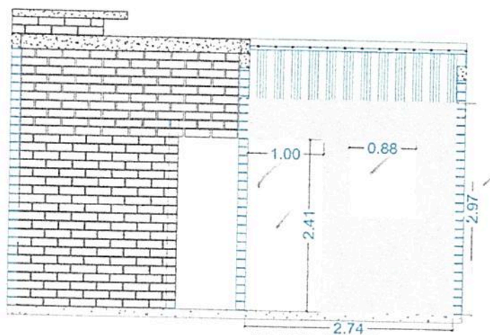
MURO EJE 5 PATIO
