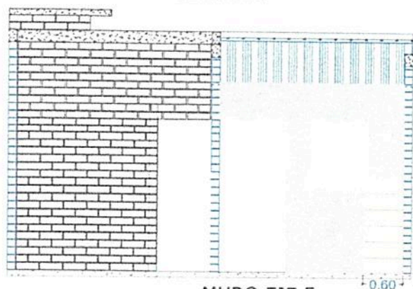
MURO EJE 5
