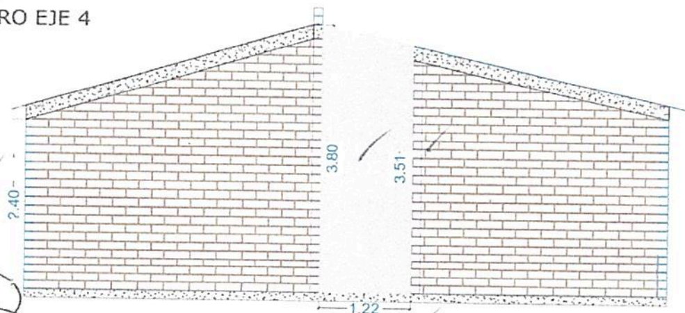
MURO EJE A
