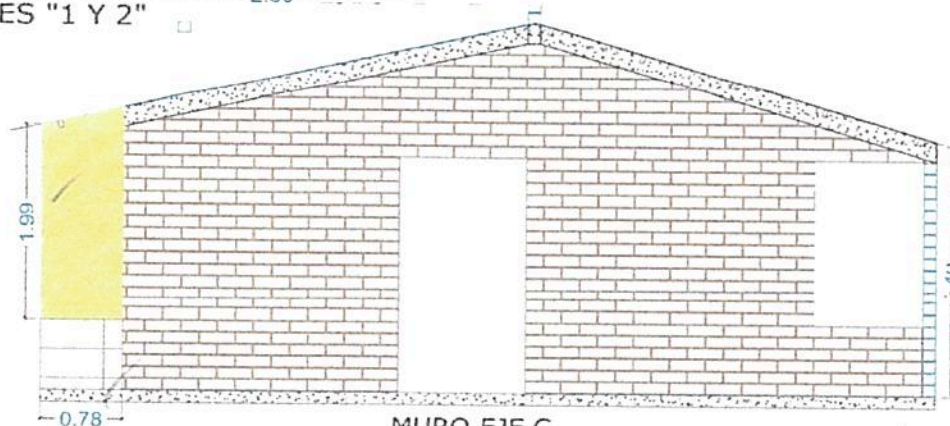
MURO EJE C
