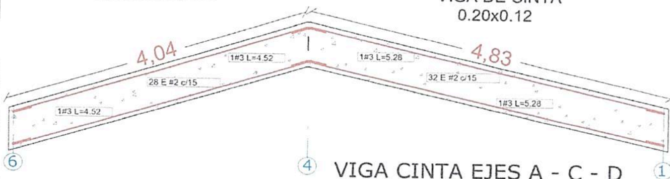
PLANTA VIGA CINTA
