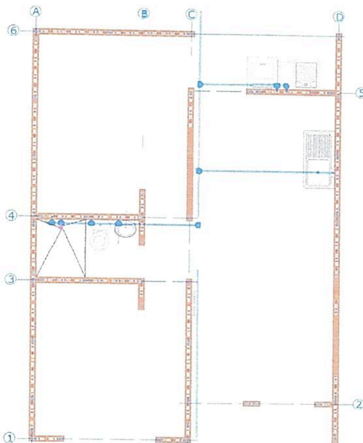
PLANTA INSTALACIONES HIDRAULICAS ESCALA 1---50
