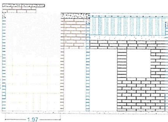
MURO EJE 4
