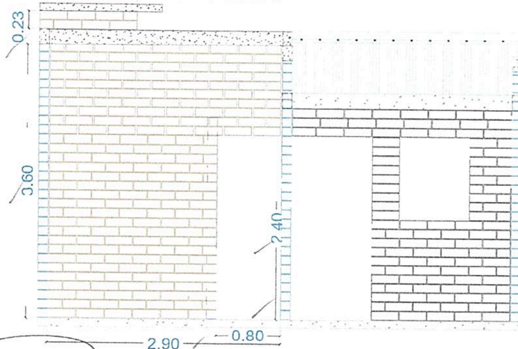
MURO EJE 4
