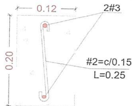
VIGA DE CINTA 0.20x0.12
