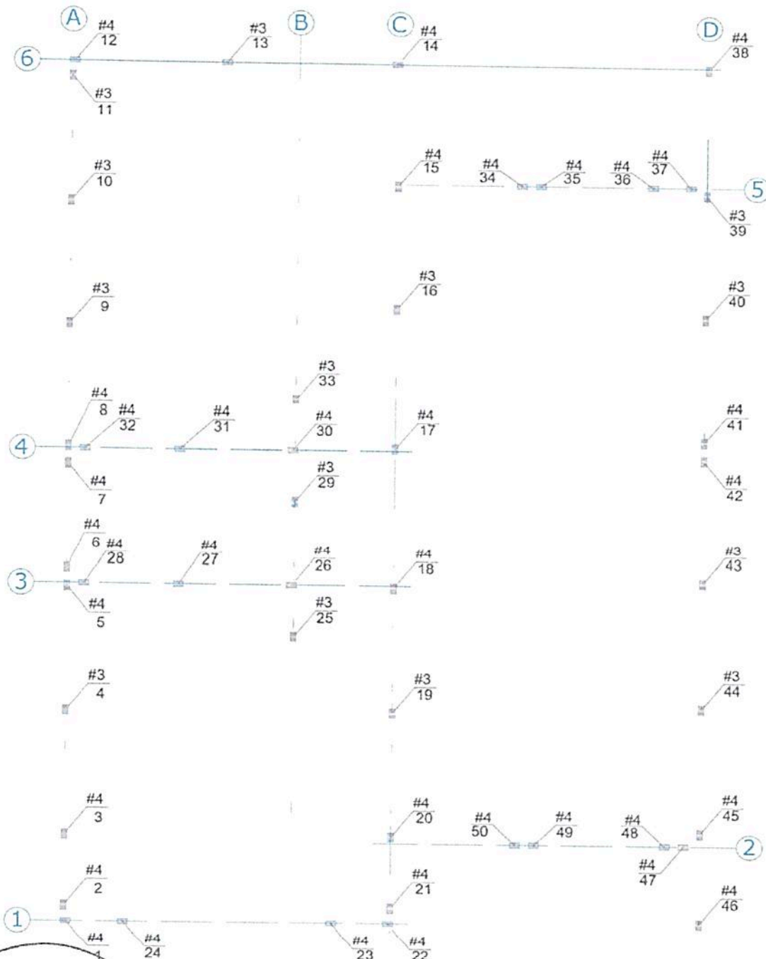
PLANTA DISTRIBUCIÓN Y REFUERZO DE MUROS DOVELAS ESCALA 1-----50
