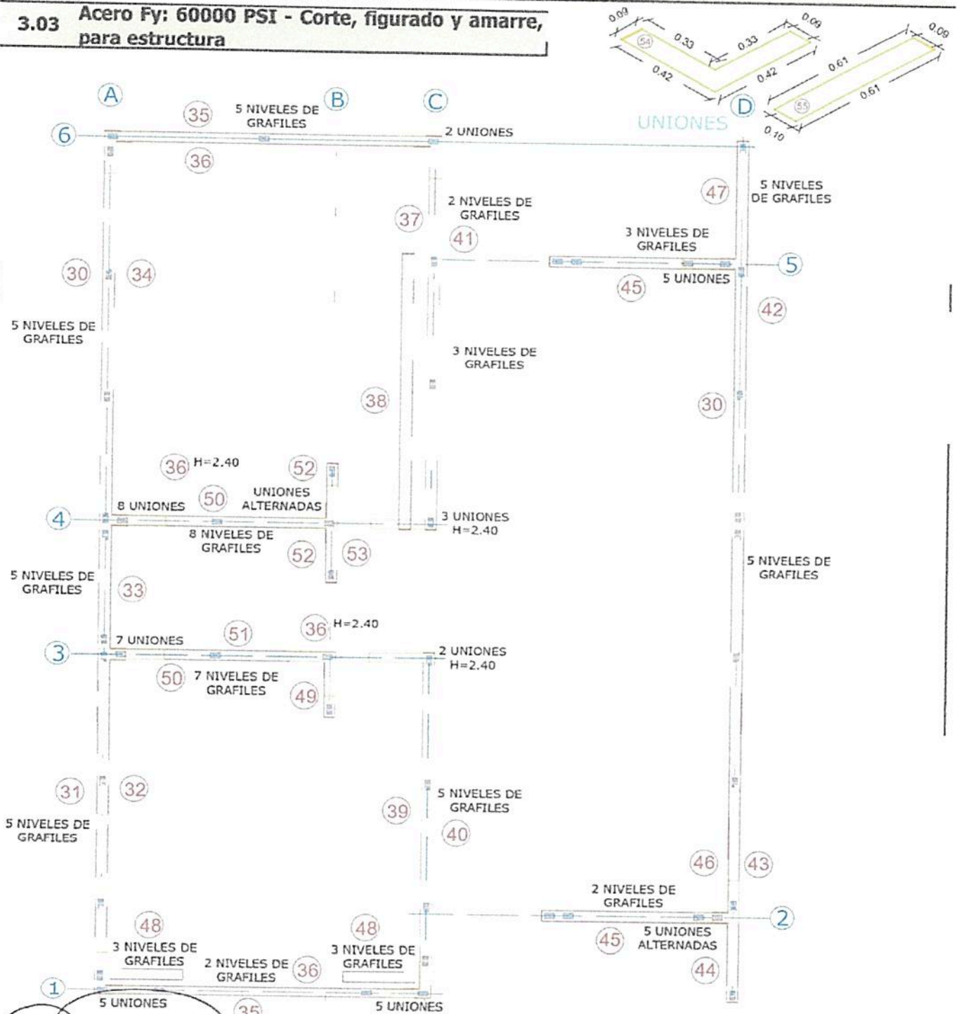
PLANTA DISTRIBUCIÓN Y REFUERZO DE MUROS GRAFILES ESCALA 1----50
