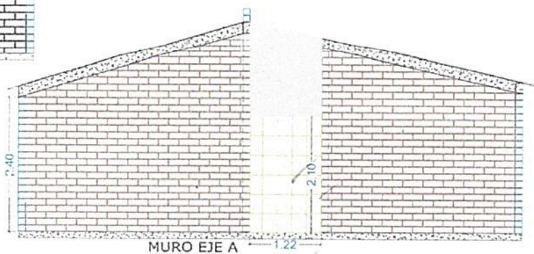
MURO EJE A
