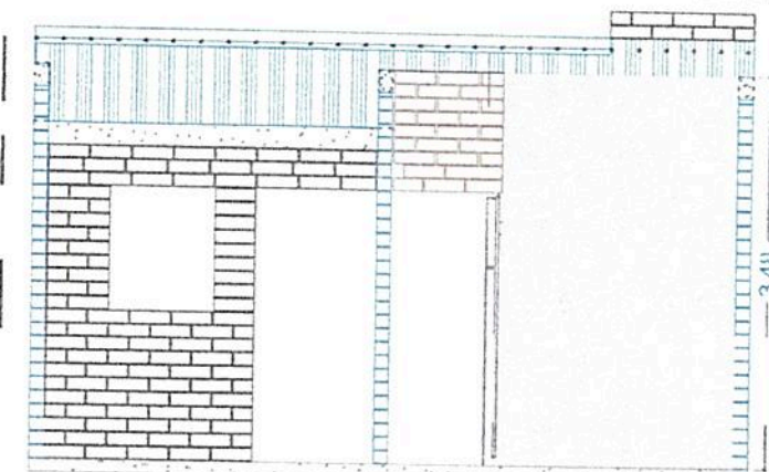
MURO EJE 3
