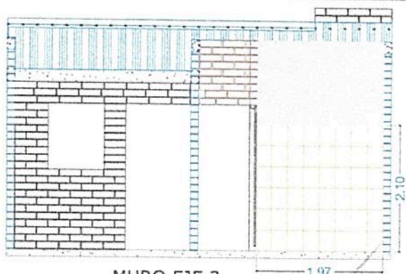
MURO EJE 3
