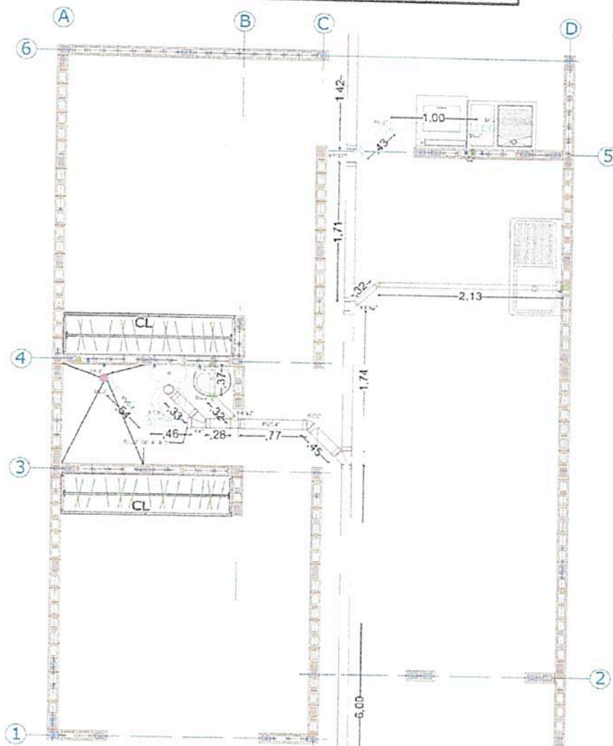
PLANTA INSTALACIONES SANITARIAS ESCALA 1----50
