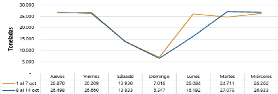
Gráfico 3. Abastecimiento diario de alimentos de las últimas dos semanas 32 mercados mayoristas 1 al 14 de octubre de 2026
