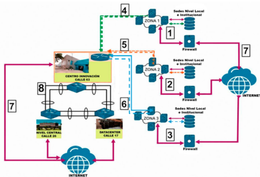
Ilustración 1 Diagrama topológico de la red.
