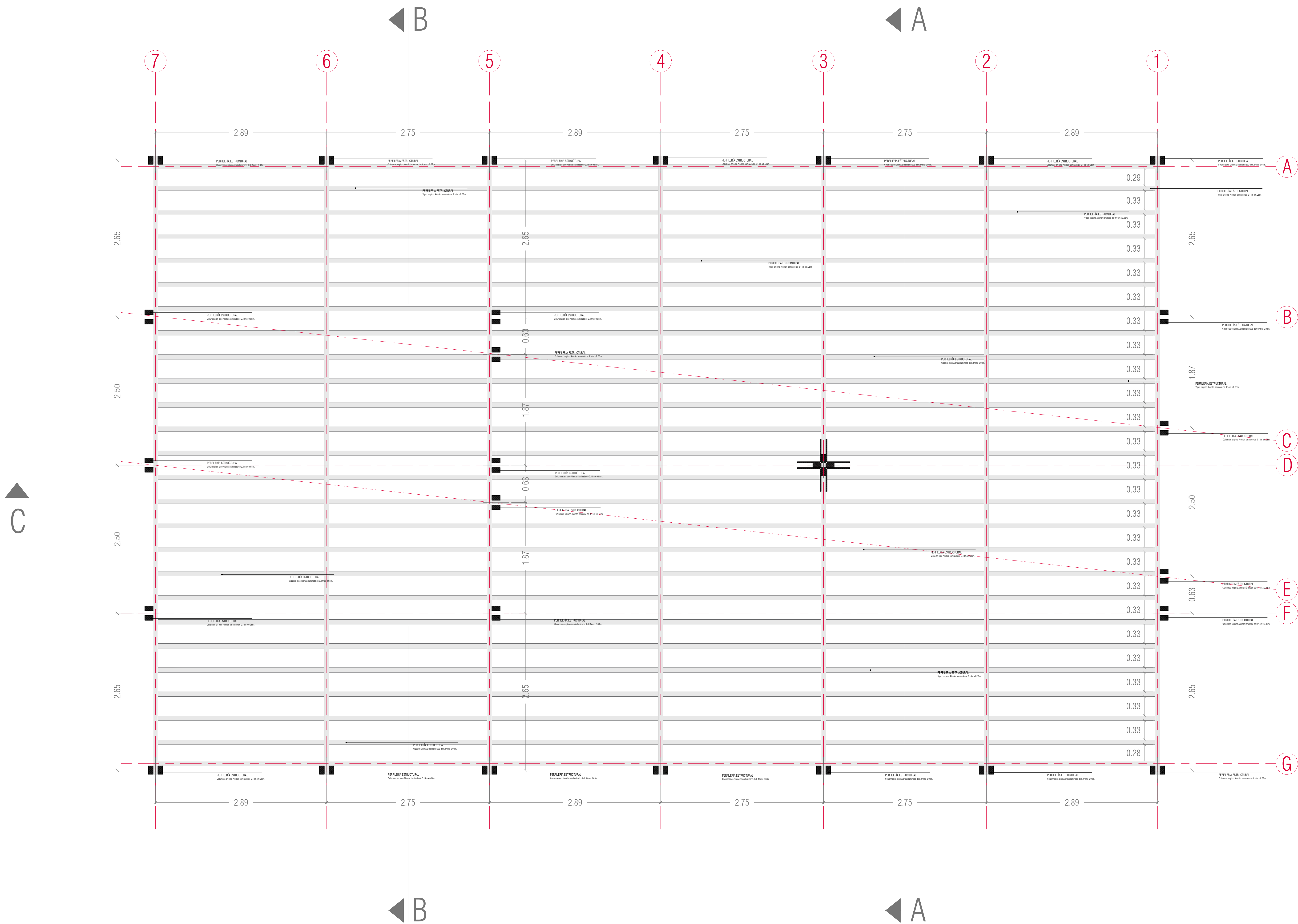
PLANTA ESTRUCTURA Entramado Inferior de Vigas Escala 1:30
