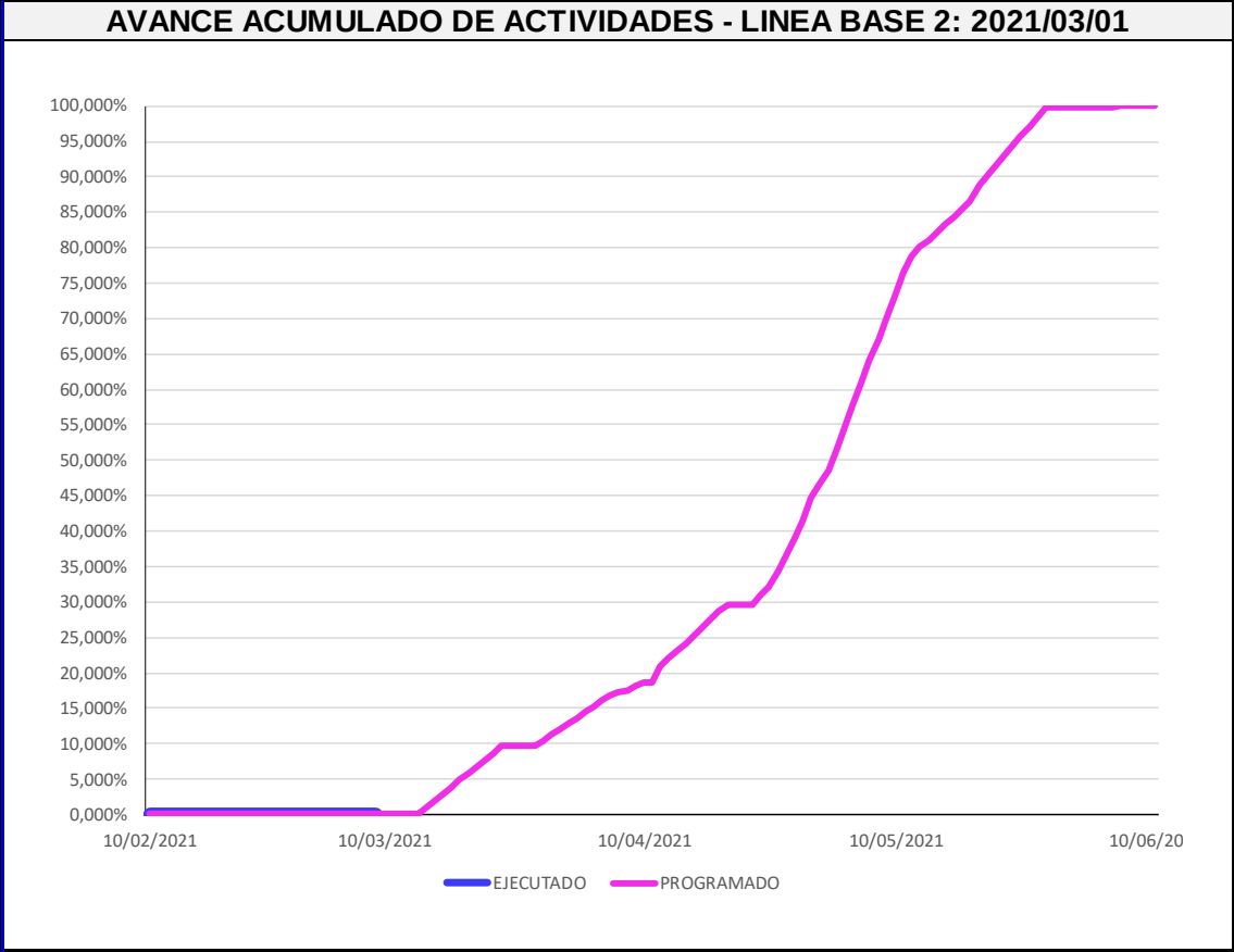
Ilustración 5: Curva S contrato 303 2020
