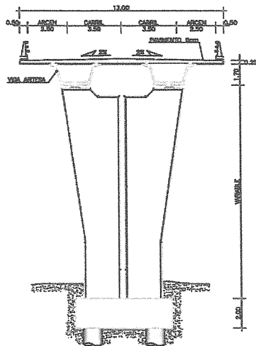
SECCIÓN TRANSVERSAL EN PUENTE SOBRE EL CAUCE ARTIFICIAL
