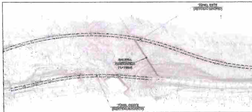
Planta de la Galería de evacuación
